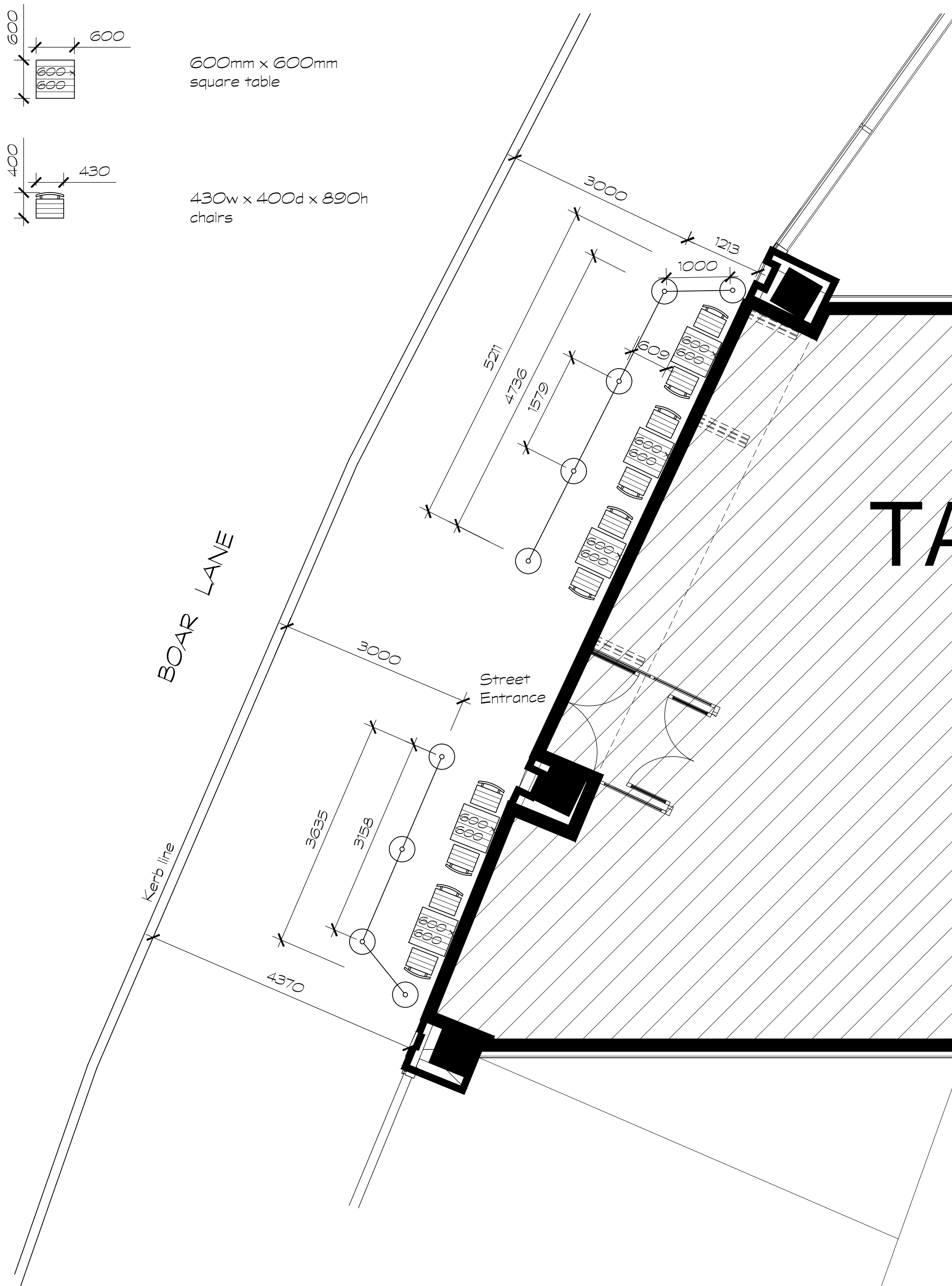
PLAN 1:50
